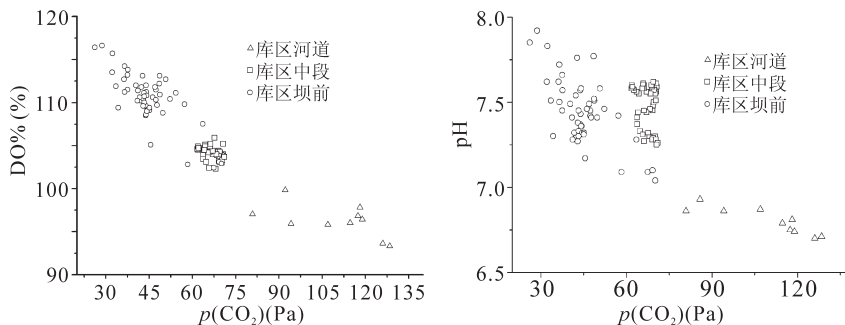
图 4 表层 p(\text{CO}_2) 与水化学参数线性关系分析图
