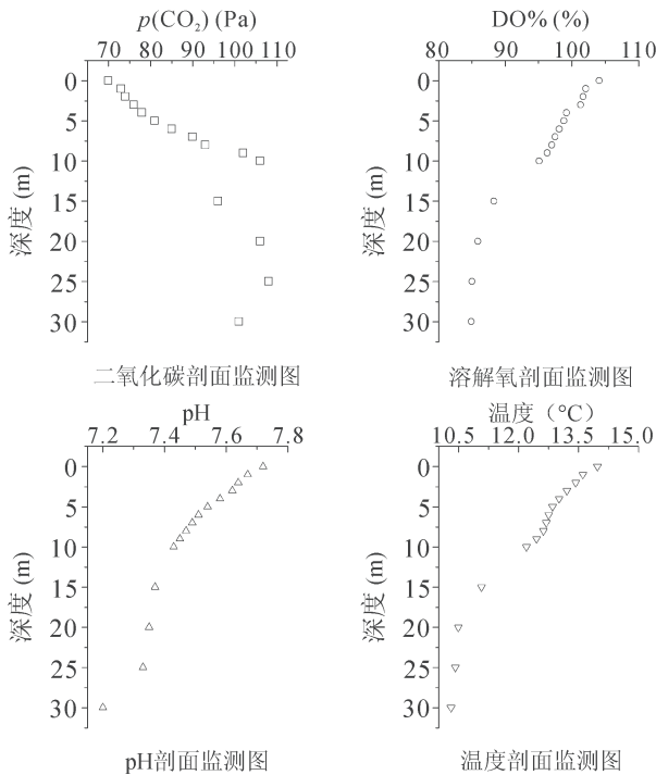
图 3 坝前剖面监测结果
