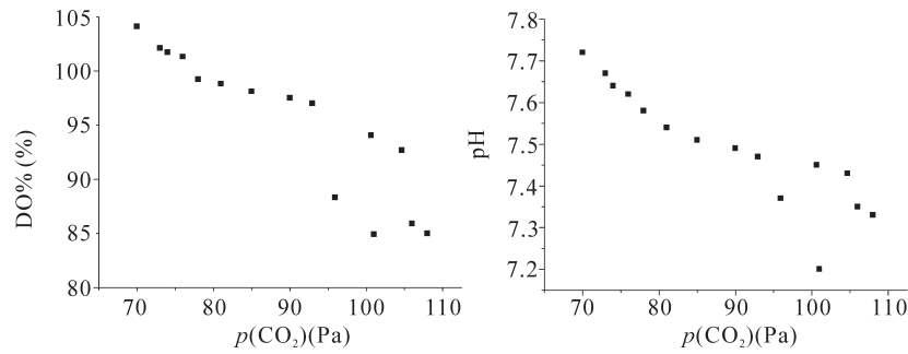
图 5 剖面 p(\text{CO}_2) 与水化学参数线性关系分析图
